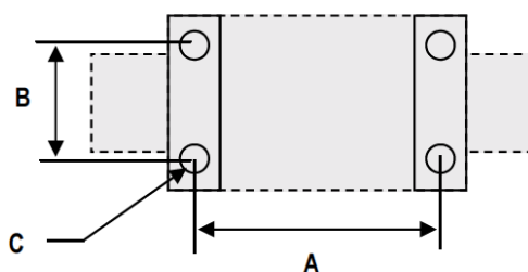
Dimensions de montage des modèles IMP4 IMP64 IMP94
