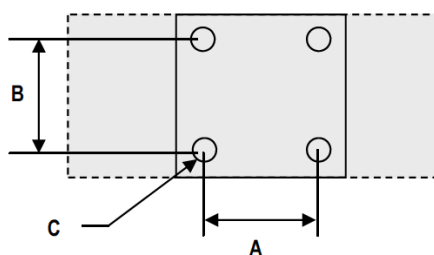
Dimensions de montage des modèles IMP4 IMP64 IMP94
